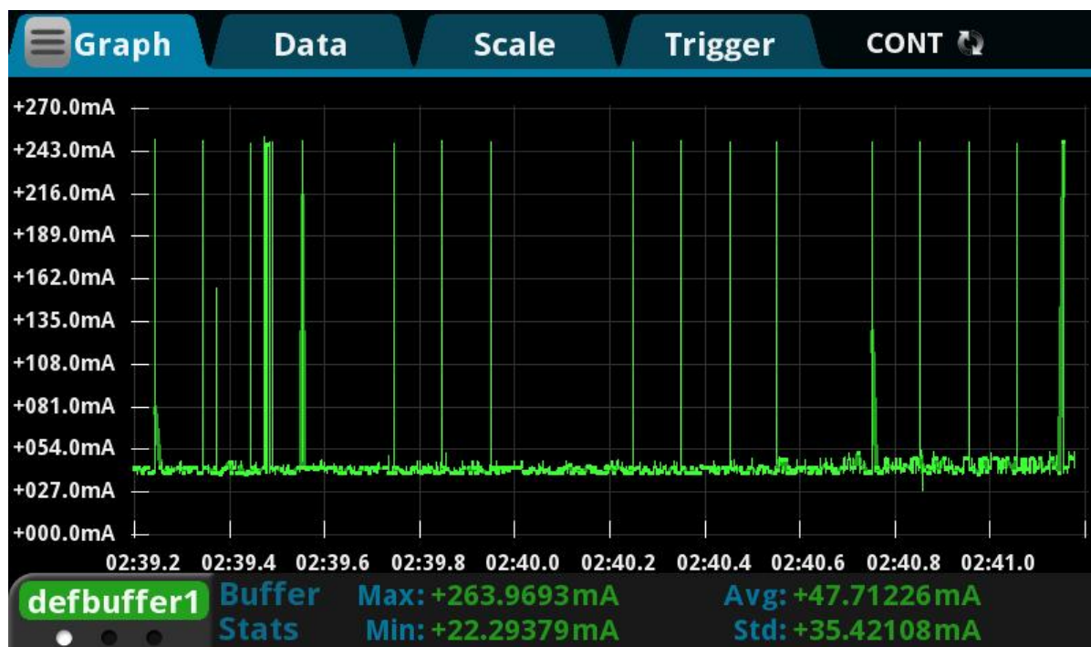
图 19 蓝牙广播开启，模块作为服务端的工作电流
