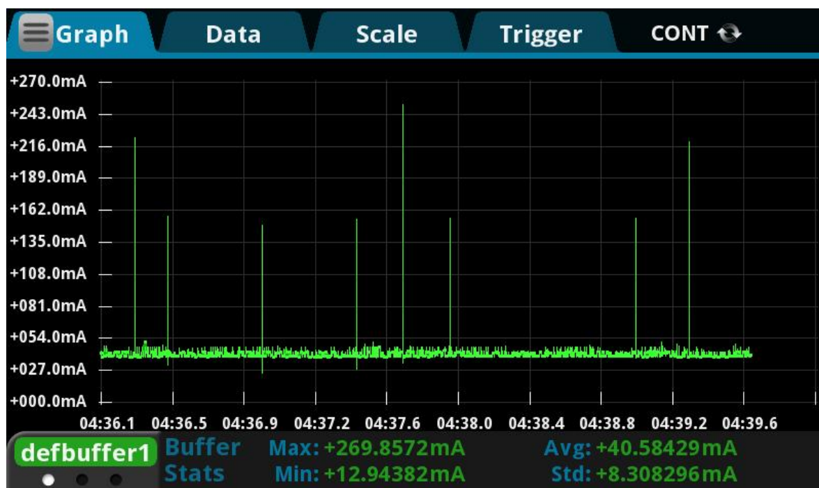
图 17 蓝牙广播开启，模块作为客户端不断尝试连接远程服务端的工作电流
