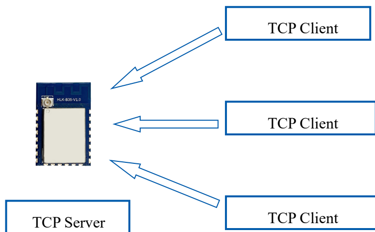
图 9 TCP Server
