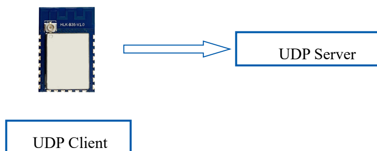
图 12 UDP Client
