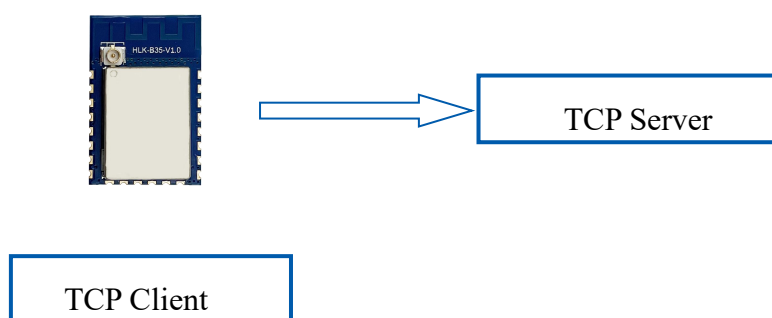
图 10 TCP Client
