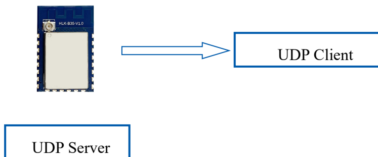
图 11 UDP Server
